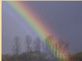
rainbow
